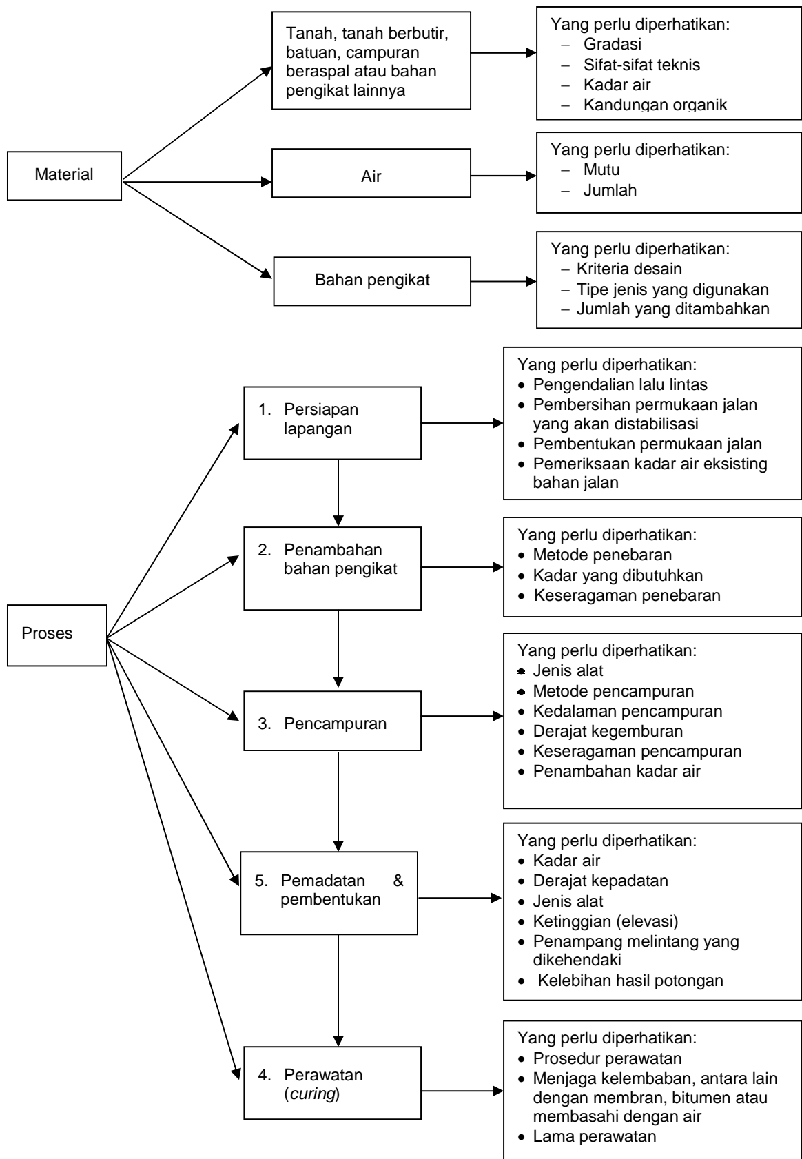
Gambar 6 - Bagan alir langkah-langkah pelaksanaan stabilisasi
