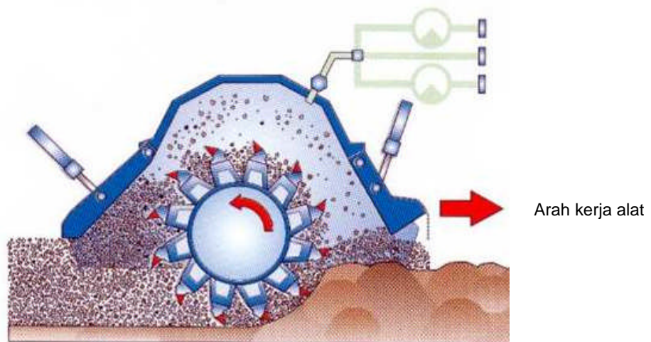
Gambar 2 - Gigi pengaduk di drum pengaduk ( miling drum )
